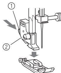
① Черная кнопка ② Адаптер прижимной лапки
