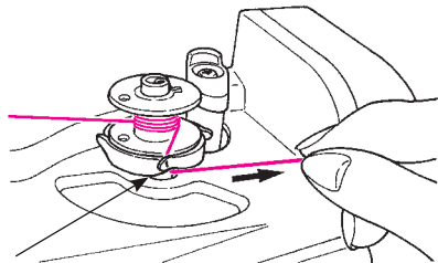
Guide (with cutter) Führung (mit Schneider) Geleider (met snijmes) направляющая (с обрезавателем)
